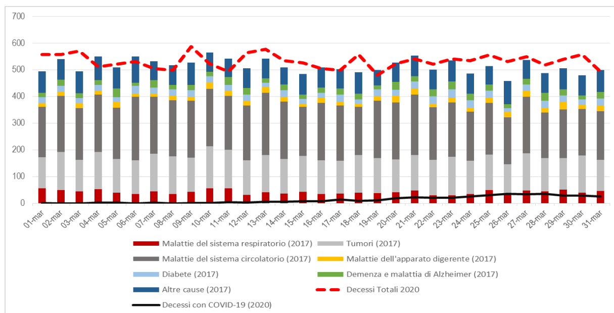
Figura 16. Confronto tra i decessi giornalieri per le principali cause iniziali di morte a marzo 2017 e i decessi con Covid-19 e per tutte le cause a marzo 2020. Area livello di diffusione Covid-19 Basso
